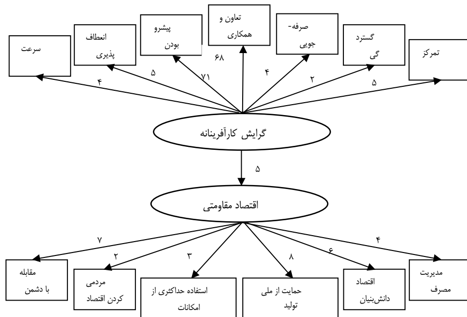
شکل ۱. مدل نهایی معادلات ساختاری به‌مراه ضرایب استاندارد
